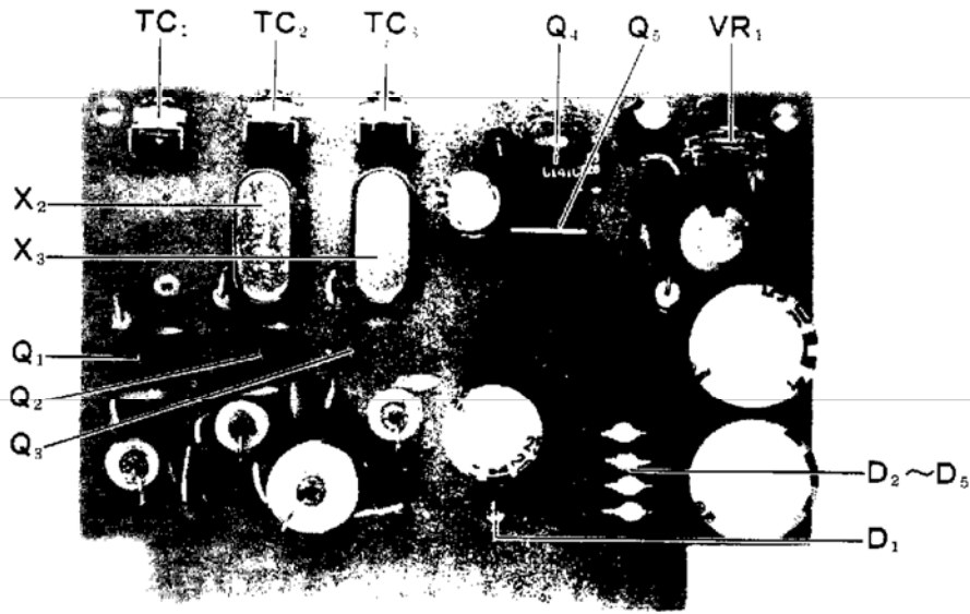
Fig. 17 REG-BFO UNIT
