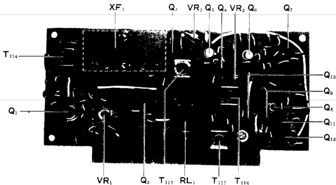
Fig. 14 NB-MIX UNIT
